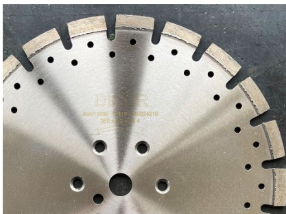
Fugentechnik, Scheibenbreite 4.3mm Asphalt für Trockenschnitt, weitverzahnt
